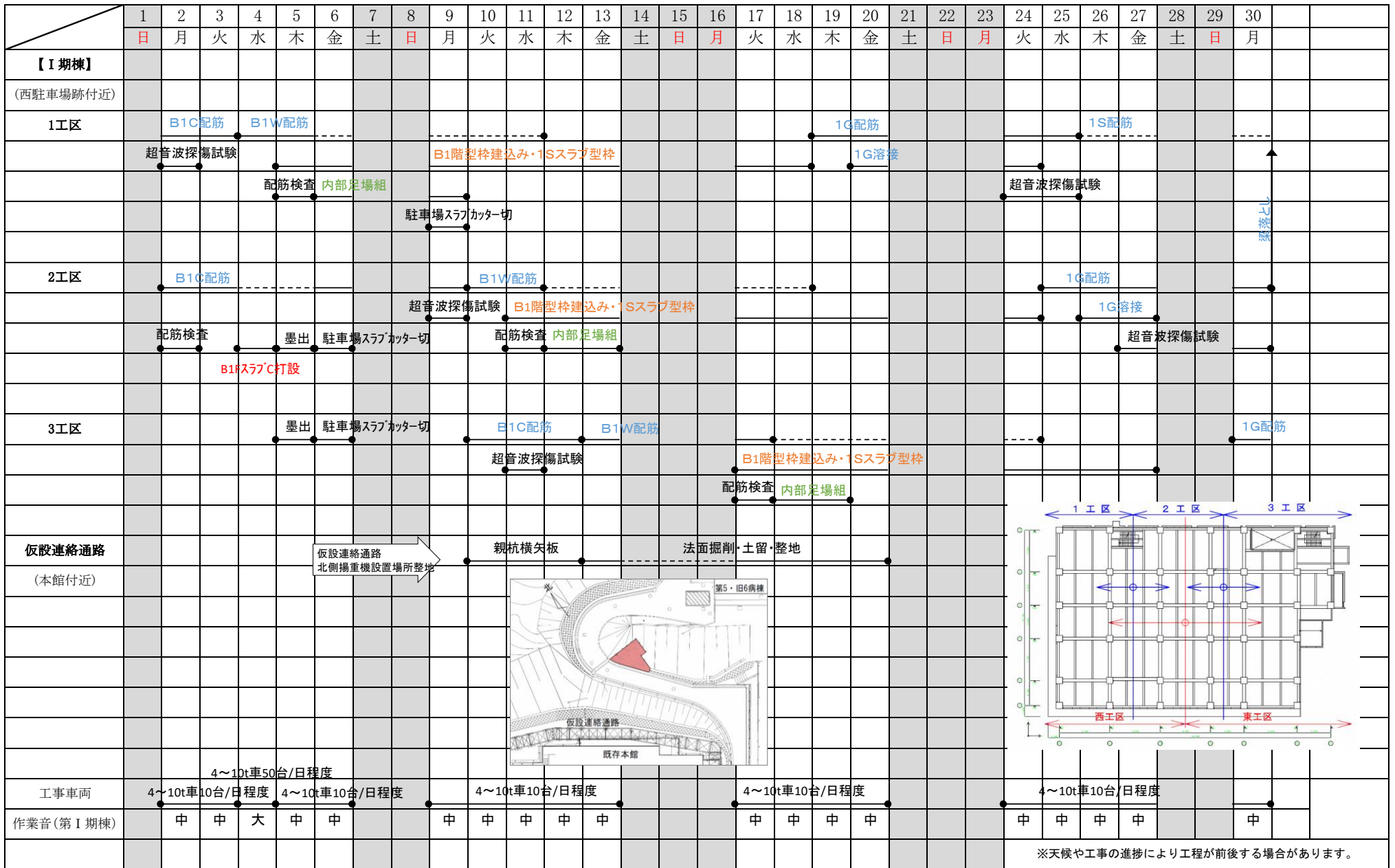
京都府立洛南病院第Ⅰ期建替工事(主体工事)(再) 令和6年9月 月間工程表
